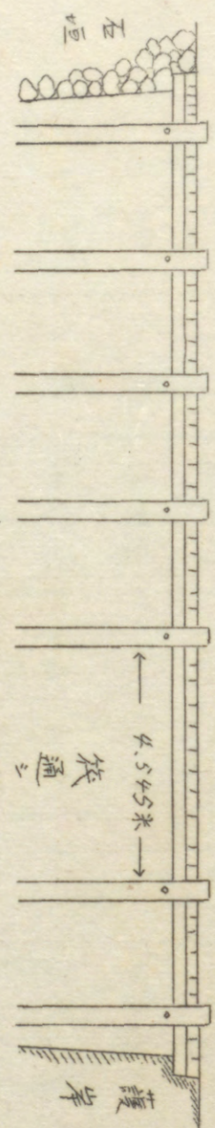
圖 造 構 橋 假 (面 側)
