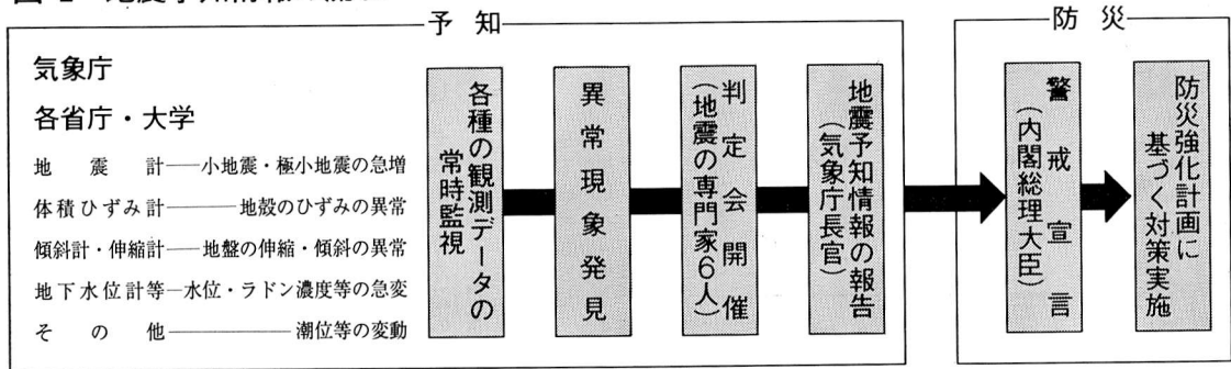
図-2 地震予知情報の流れ
