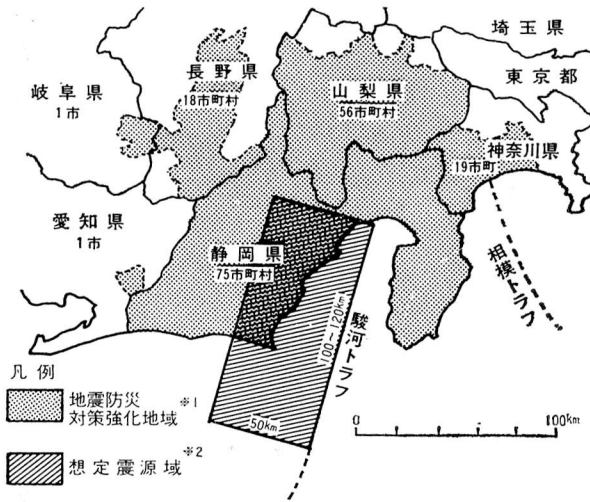
図-1 地震防災対策強化地域及び想定震源域
