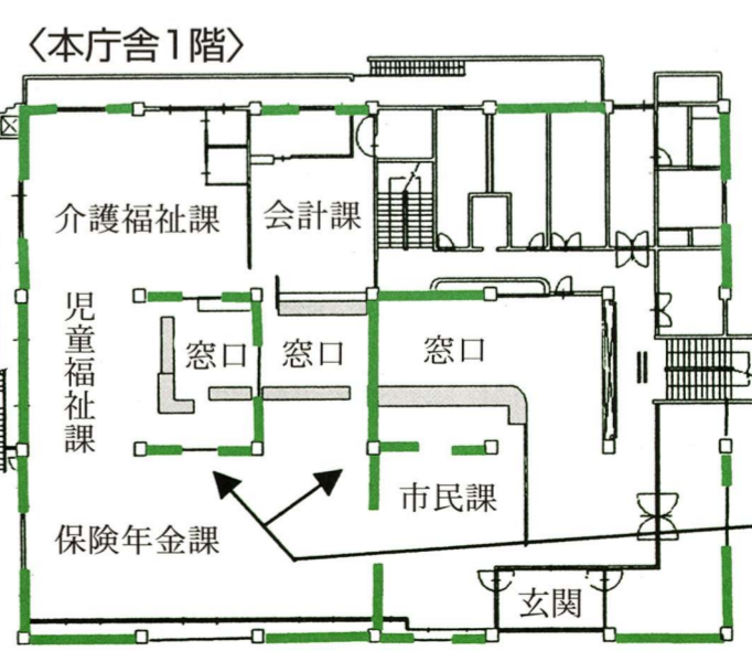
図1 耐震補強壁設置箇所(一部分)
