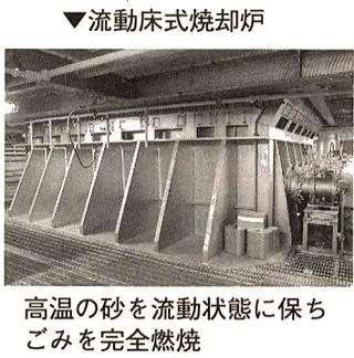
流動床式焼却炉
