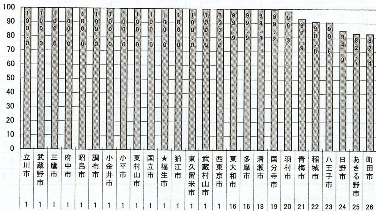
4-2. グラフ 下水道普及率（平成16年度） 単位：%
