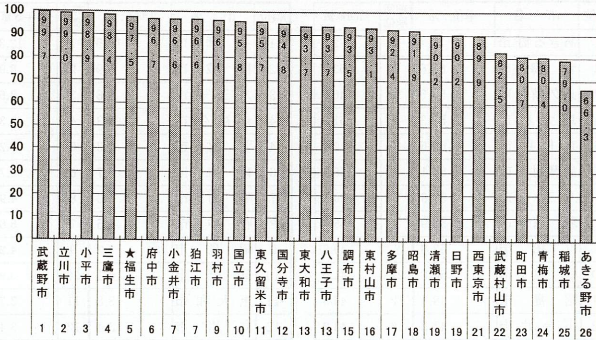
4-1. グラフ 道路舗装率（平成16年度） 単位：%
